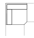
angolo da 108 L. 108 P. 108 H. 83
