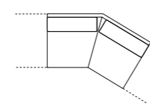
angolo sagomato da 181x131 L. 181 P. 131 H. 83
