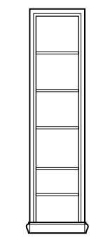
Art. 5935/D Colonna a giorno L. 64 P. 42 H. 217
