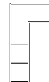
Art. 7354/D Pensile libreria 3 vani Sx L. 66,5 P. 36 H. 118 L. 29,5 H. 88,5 angolo 37
