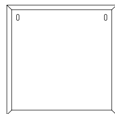
Art. 4980/D Pensile 1 vano L. 59 P. 36 H. 59
