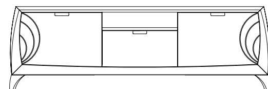
Art. 6149/D Base 3 cestoni con incisioni e vano L. 189 P. 57 H. 60
