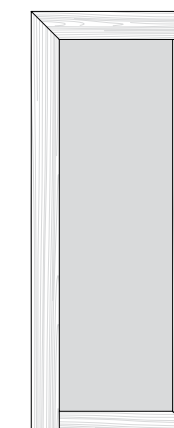
Art. 6228/D Anta telaio vasistas Vert. Sx vetro Per argenteria L. 58,6 H. 153,5
