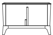
Art. 7312/D Sx - Art. 7313/D Dx Base 1c. liscio con man. legno e piedini L. 83,5 P. 56 H. 54,3
