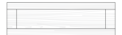
Art. 5019/D Anta orizzontale telaio L. 117,6 H. 36,6
