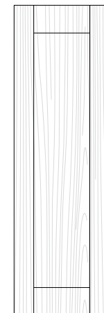
Art. 5009/D Anta telaio vert. L. 36,6 H. 117,6
