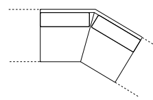
angolo sagomato da 181 L. 181 P. 131 H. 83
