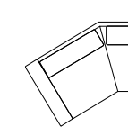
terminale sagomato da 197 dx/sx L. 197 P. 141 H. 83
