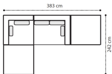
PM/12 Usx + Jdx + Pouff121 + Pouff121
