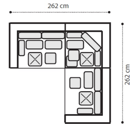
PAG.27 PIUMA Jsx + U + Jdx + 3A + 4B + 4C note: Cuschions C, E in cat. E 262 x 262 x H. 63 cm
