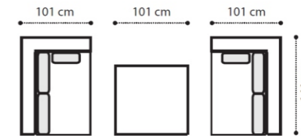
PM/10 Wsx + Pouff101 + Wdx
