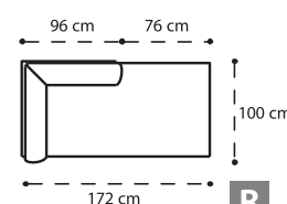
PENISOLA CONTENITORE (R) STORAGE ELEMENT (R) ШЕЗЛОНГ С КОРОБОМ (R) 1.62 m 3 – 68.5 kg.
