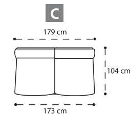
DIVANO 3 POSTI CENTRALE (C) CENTRAL 3 SEATER ELEMENT (C) ЦЕНТРАЛЬНЫЙ 3 –ЕХ МЕСТНЫЙ ЭЛЕМЕНТ (C)
