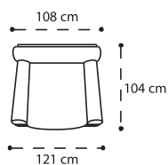
POLTRONA ARMCHAIR КРЕСЛО 1.19 m 3 – 48 kg.
