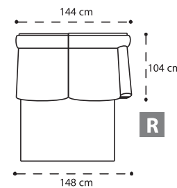
DIVANO 2 POSTI LATERALE (R) + LETTO 2 SEATER SIDE ELEMENT (R) + BED ДИВАН 2-ЕХ МЕСТНЫЙ БОКОВОЙ (R) + КРОВАТЬ 1.67 m 3 – 72 kg. (Mattress size 90 x 180 cm)
