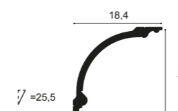
C338 BA'ROCK 200 x 18,4 x 18,4 cm Purotouch ®
