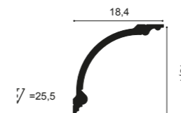
C338A BA'ROCK 200 x 18,4 x 18,4 cm Purotouch ®
