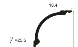
C338B BA'ROCK 200 x 18,4 x 18,4 cm Purotouch ®
