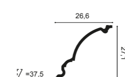
C336 BA'ROCK 200 x 27,1 x 26,6 cm Purotouch ®
