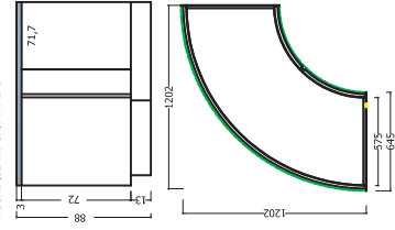
ISOLA CIRCOLARE TIPO "D" 1202 X 1224 ROUND ISLAND UNIT TYPE "D"
