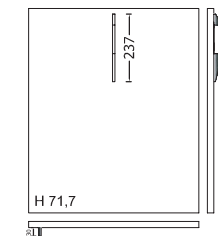
COLONNA ANTA CESTELLO ESTRAIBILE COLUMN PULL-OUT BASKET DRAWER DOOR
