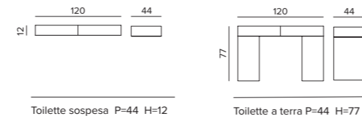
Toilette sospesa P=44 H=12
