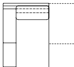
penisola da 106x150 dx/sx L. 106 P. 150 H. 82
