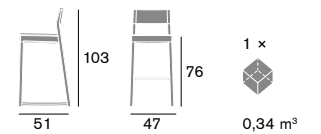
Linea 1013 SG Dimensioni / Sizes
