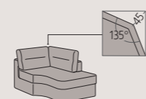
Divano laterale dx/sx L 185 P 93 H 100 - Letto
